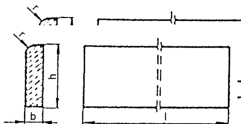
Rysunek 2. Kształt betonowego obrzeża chodnikowego
